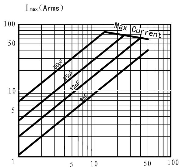
频率曲线 (MHz) U_{pw}=25kV
